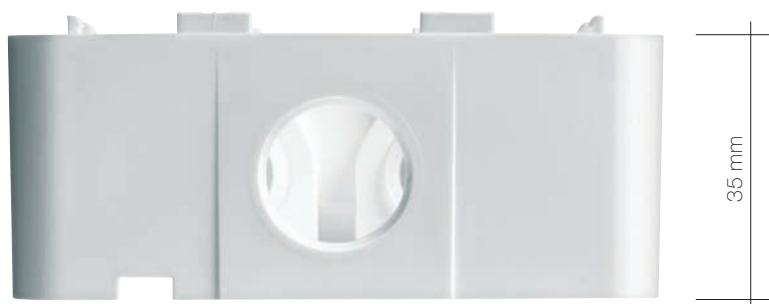
Querschnitt NAP-Gehäuse 35 mm
