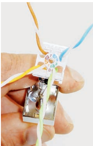
Mehr Platz im Deckel: eindeutige Aderzuordnung im Aderorganisator.
