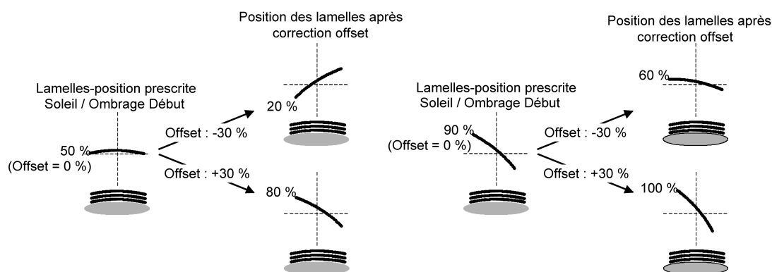
Figure 21: Mode de fonctionnement de l'offset de lamelles comme exemple (particulièrement pour type de lamelles 1/type de lamelles 2 équivalent en substance)
