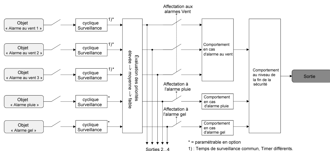
Figure 15: Schéma fonctionnel des fonctions de sécurité orientées canal
