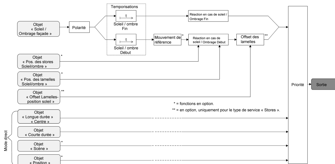
Figure 18: Schéma fonctionnel de la protection solaire simple
