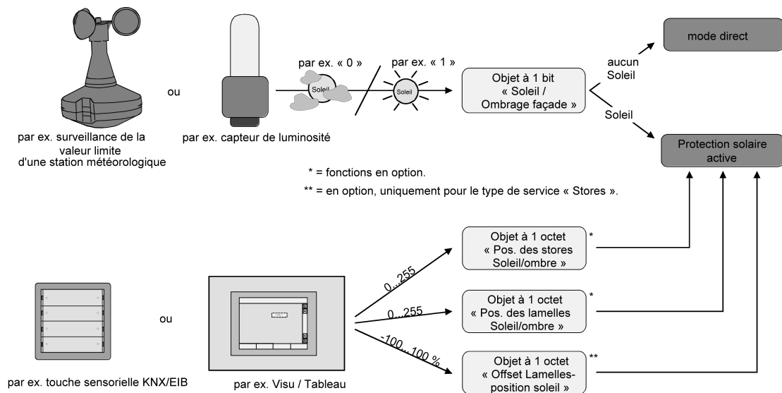
Figure 17: Schéma de principe de la protection solaire simple
