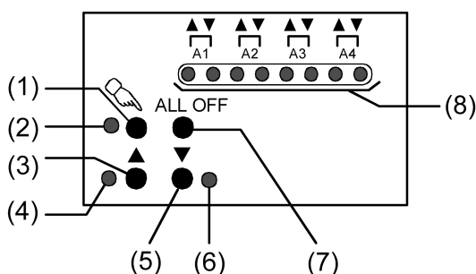
Figure 5: Éléments de commande et d'affichage de la commande manuelle à l'avant de l'appareil
