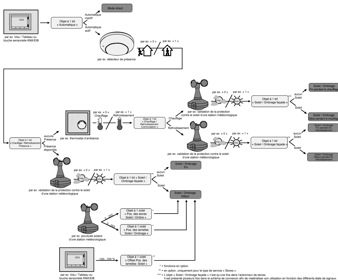
Figure 22: Schéma de principe du chauffage/refroidissement automatique (pour simplifier sans fonctions de blocage du mode automatique ou du mode direct)
