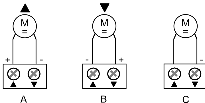
Figure 3: Polarité au niveau des moteurs d'entraînement selon le sens de mouvement (A et B) et lorsque l'entraînement est à l'arrêt (C).
