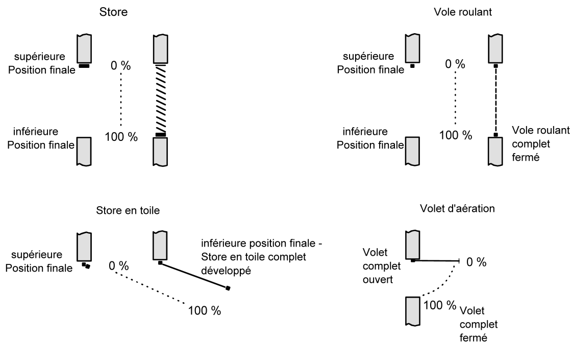
Figure 11: Définition de la position en fonction du type d'entraînement
