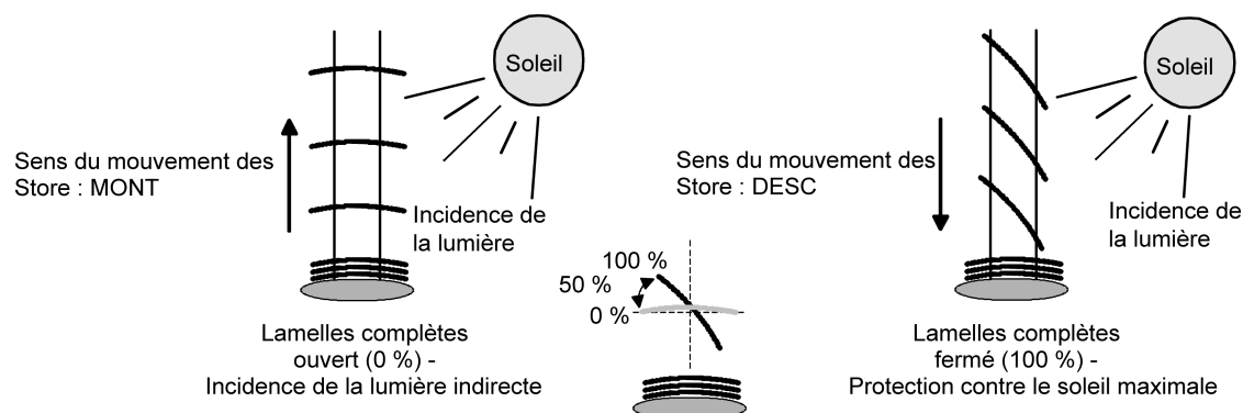
Figure 10: Type 2 - Stores à lamelles avec position des lamelles en biais et droite
