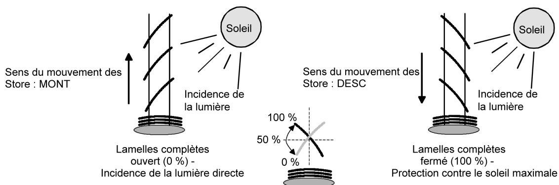
Figure 9: Type 1 - Stores à lamelles avec position des lamelles en biais dans les deux sens de mouvement
