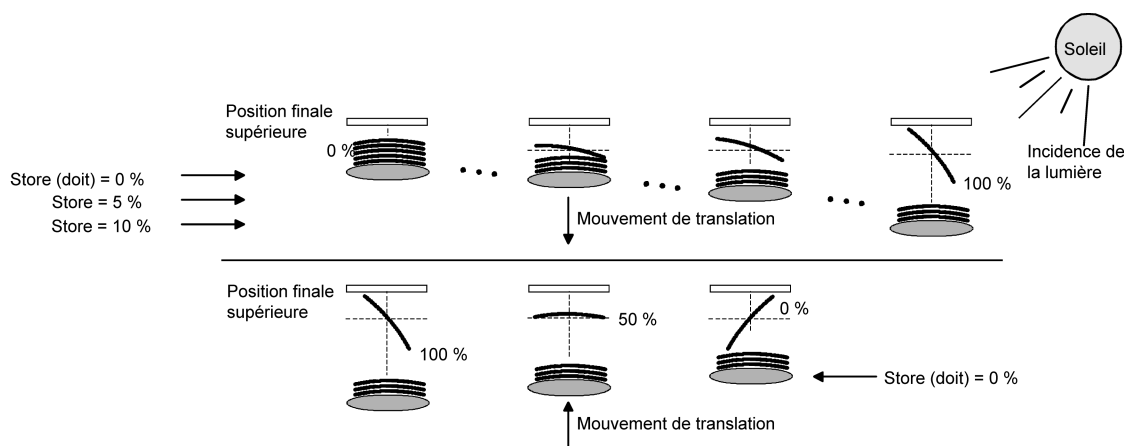
Figure 13: Exemple de positionnement des lamelles pour une position de store en fin de course supérieure (Particulièrement pour type de lamelles 1.)
