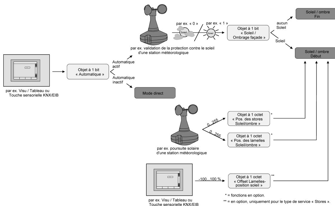
Figure 19: Schéma de principe de la protection solaire étendue (pour simplifier sans fonctions de blocage)
