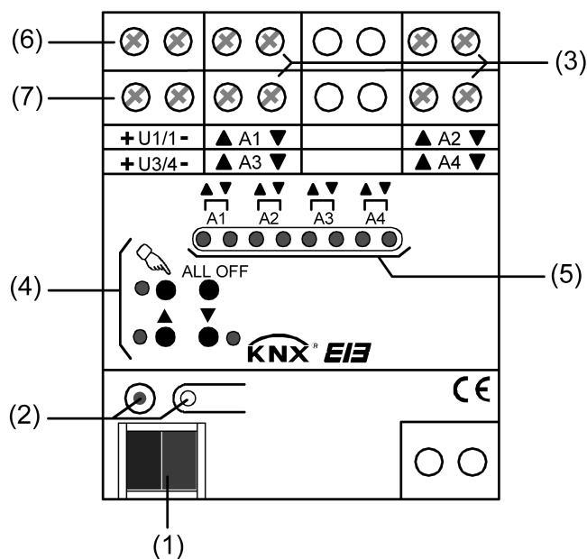
Figure 1: Conception de l'appareillage
