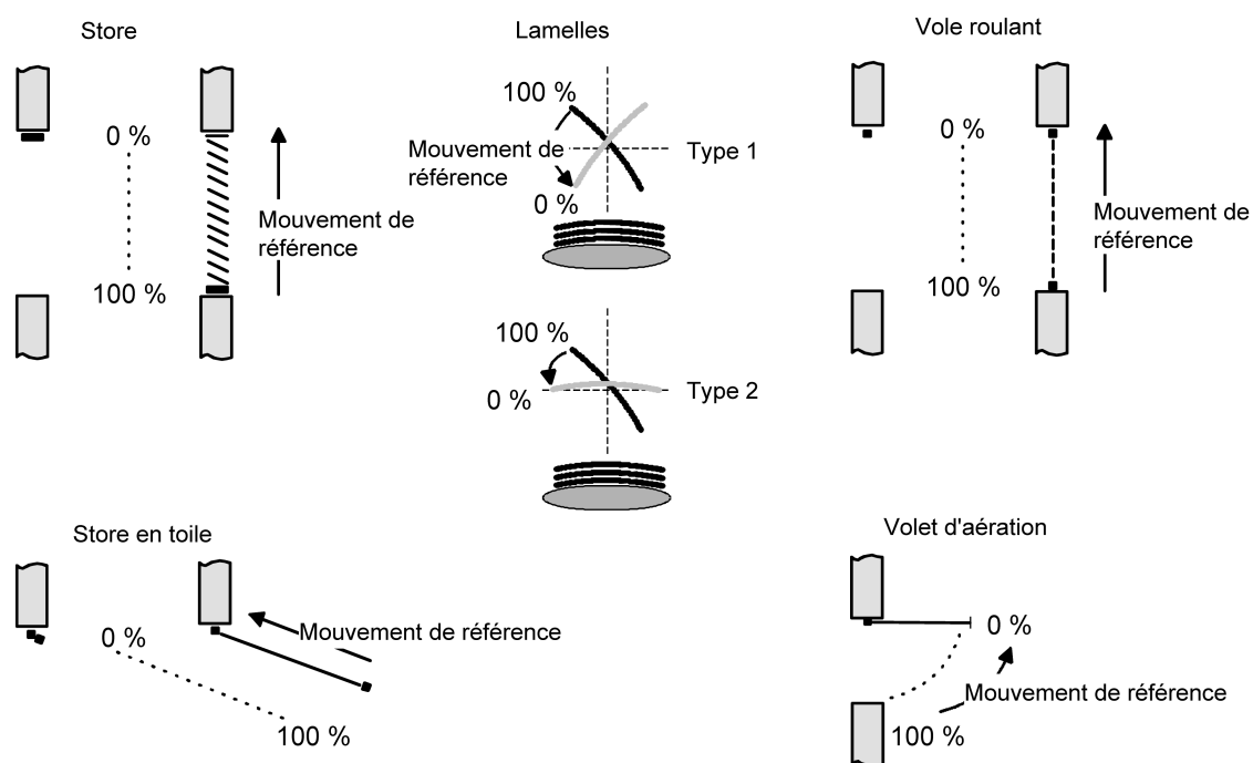
Figure 14: Course de référence
