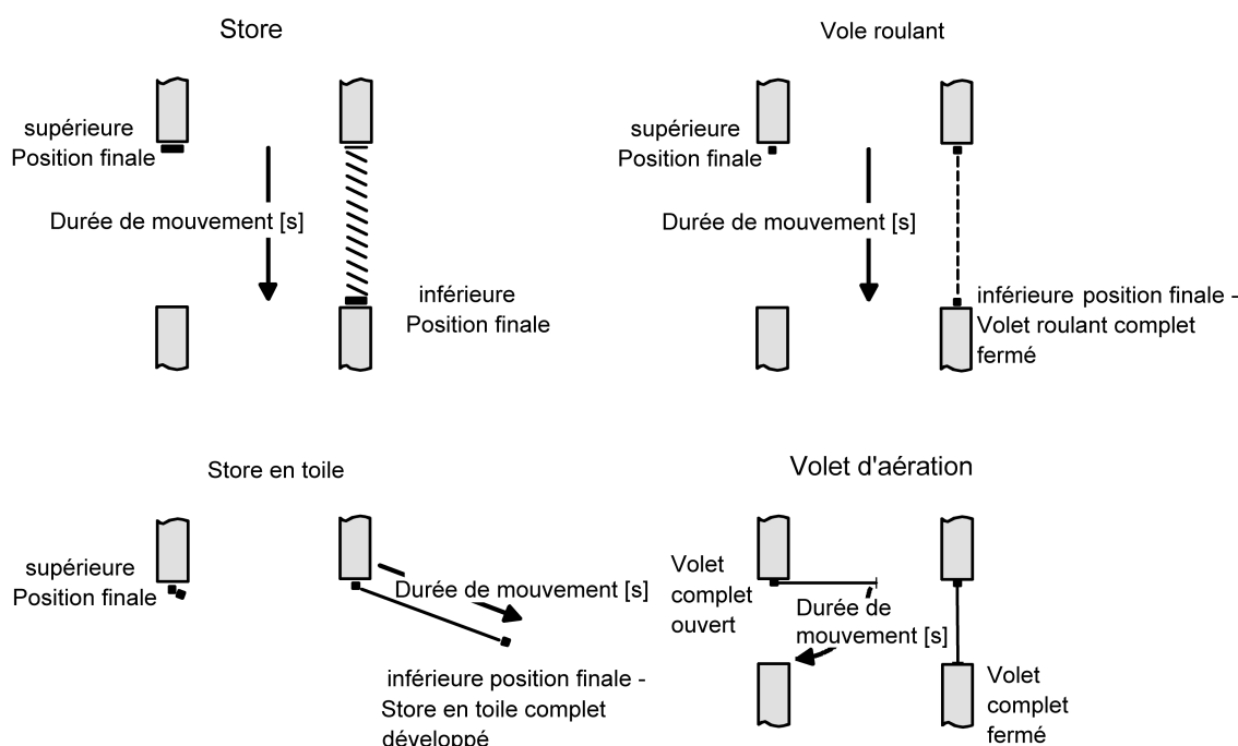
Figure 8: Détermination de la durée de mouvement en fonction du type d'entraînement
