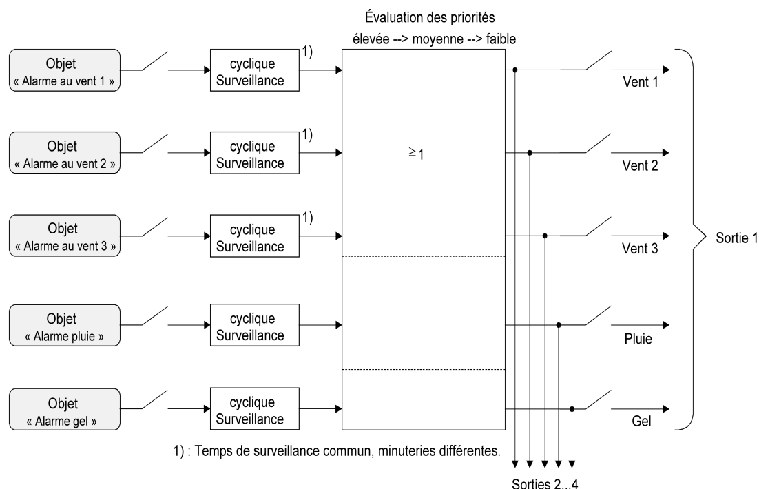
Figure 7: Schéma fonctionnel des fonctions de sécurité
