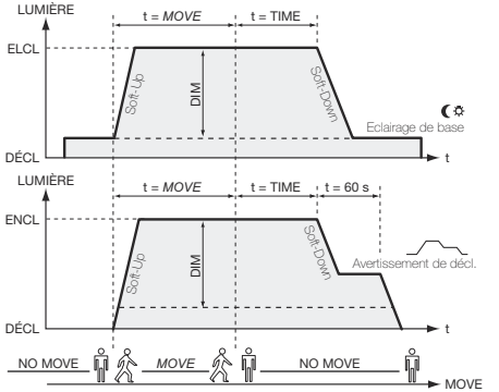
fig. 2 Eclairage de base / Avertissement de décl.
