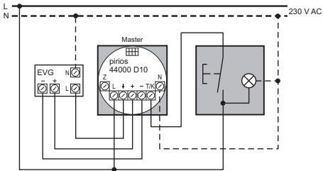
fig. 1 Fonction de poussoir Encl./Eco-Décl Il est possible de raccorder jusqu'à 10 appareils au Master (p.ex. 3 Slaves et 7 poussoirs zeption!) Le nombre de poussoirs classiques est illimité. La longueur de la liaison aux poussoirs ne doit pas dépasser 100 m.
