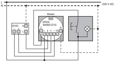
fig. 3 Fonction de poussoir Redéclenchement Tous les appareils pirios associés doivent être alimentés par le même conducteur de phase et protégés par le même groupe de fusibles.
