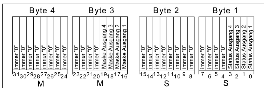
Bild 12: Struktur des Objekts "23" der Sammelrückmeldung für die Ausgänge 1 ... 4
