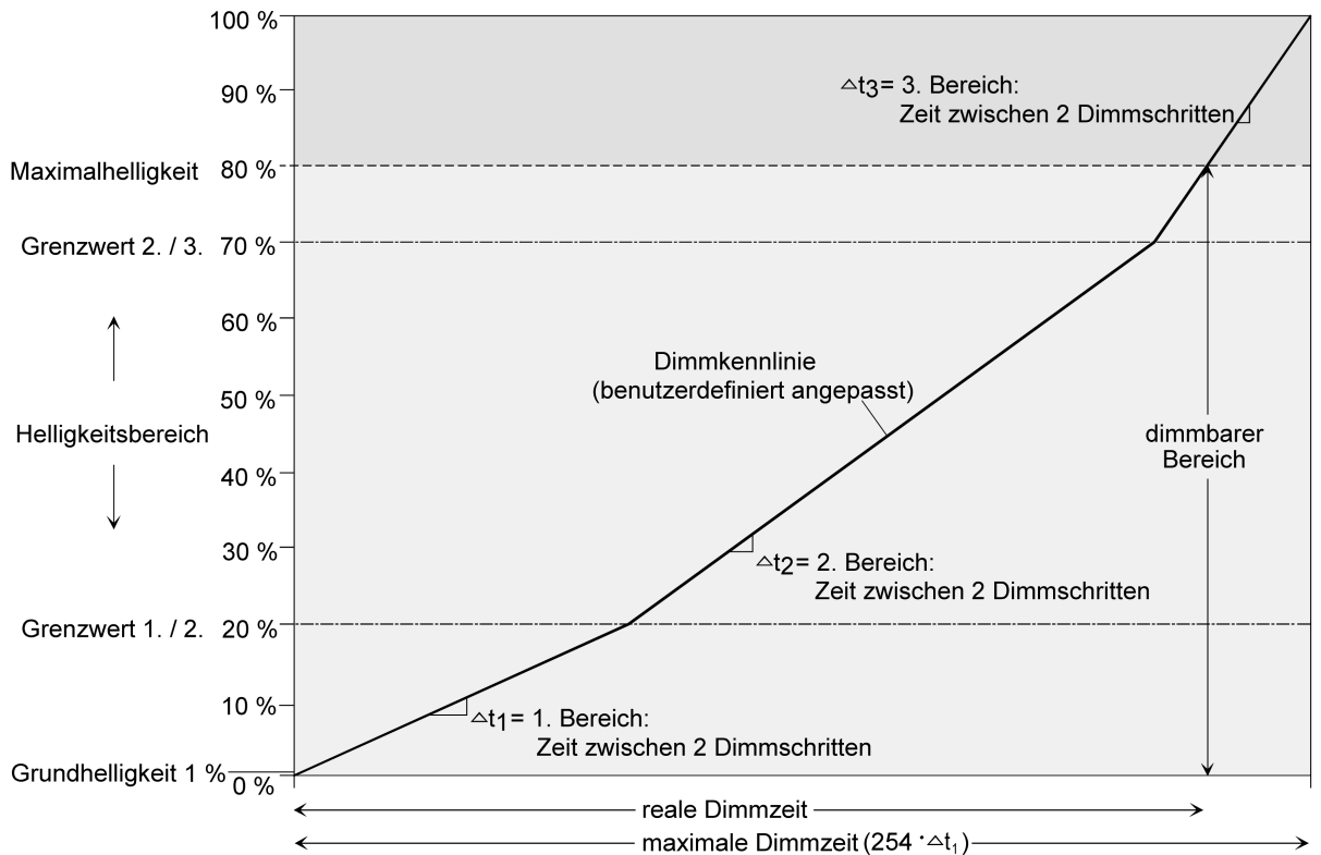
Bild 8: Benutzerdefinierte Dimmkennlinie als Beispiel mit Grundhelligkeit und Maximalhelligkeit
