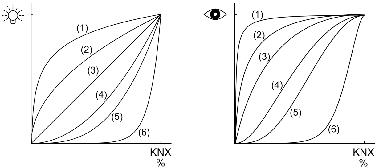
Bild 5: Dimmkennlinien im Wertebereich
