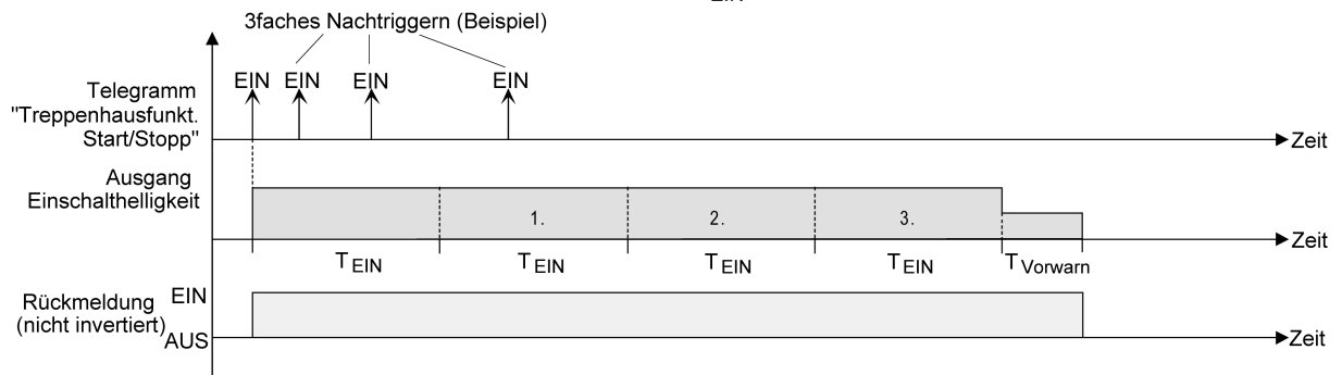
Bild 23: Zeitverlängerung der Treppenhausfunktion
