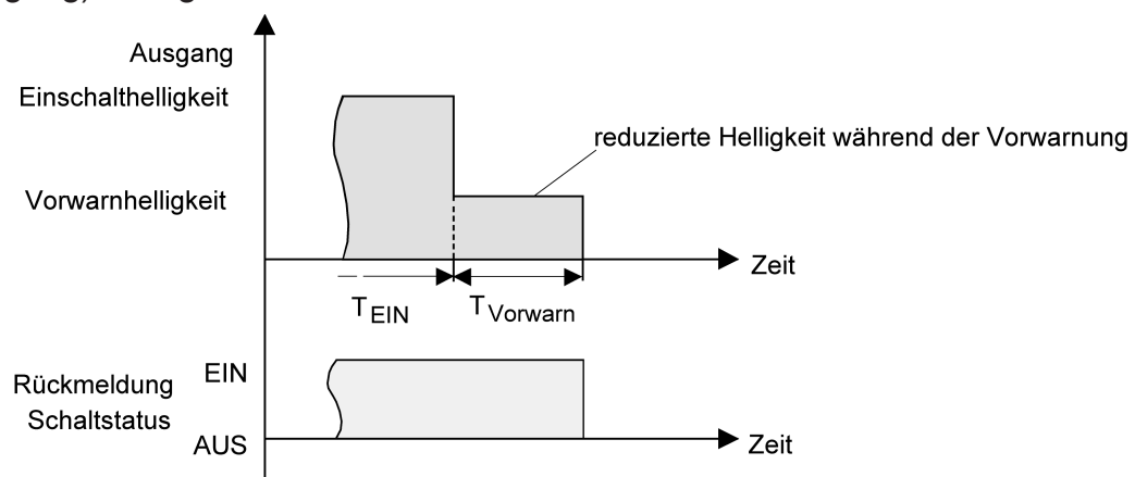
Bild 19: Die Vorwarnfunktion der Treppenhausfunktion ohne Soft-AUS-Funktion
