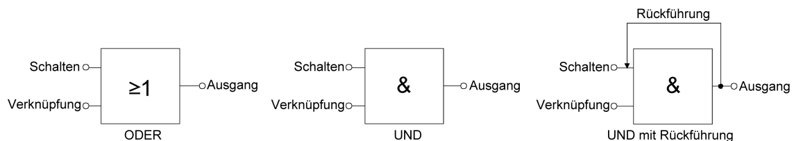
Bild 24: Verknüpfungsarten der Verknüpfungsfunktion
