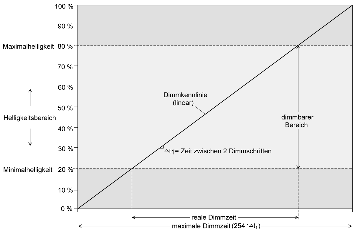
Bild 7: Lineare Dimmkennlinie als Beispiel mit Minimalhelligkeit > 0 % und Maximalhelligkeit
