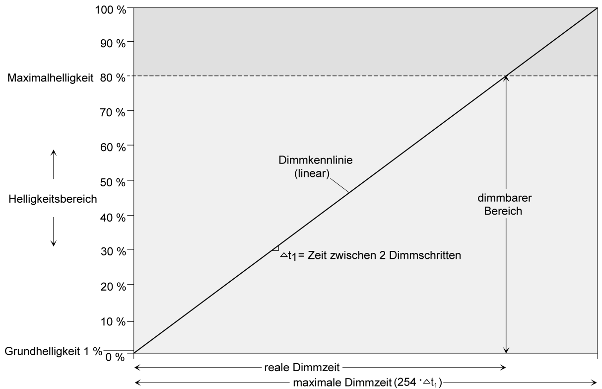
Bild 6: Lineare Dimmkennlinie als Beispiel mit Grundhelligkeit und Maximalhelligkeit
