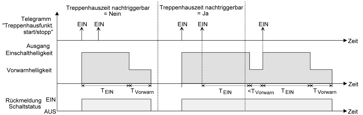
Bild 15: Einschaltverhalten der Treppenhausfunktion ohne Soft-Funktionen
