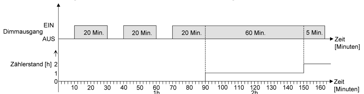
Bild 25: Funktionsweise des Betriebsstundenzählers (am Beispiel gezählter Stunden)
