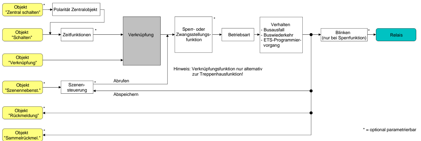
Fig. 19: Funktionsschaltbild der Verknüpfungsfunktion
