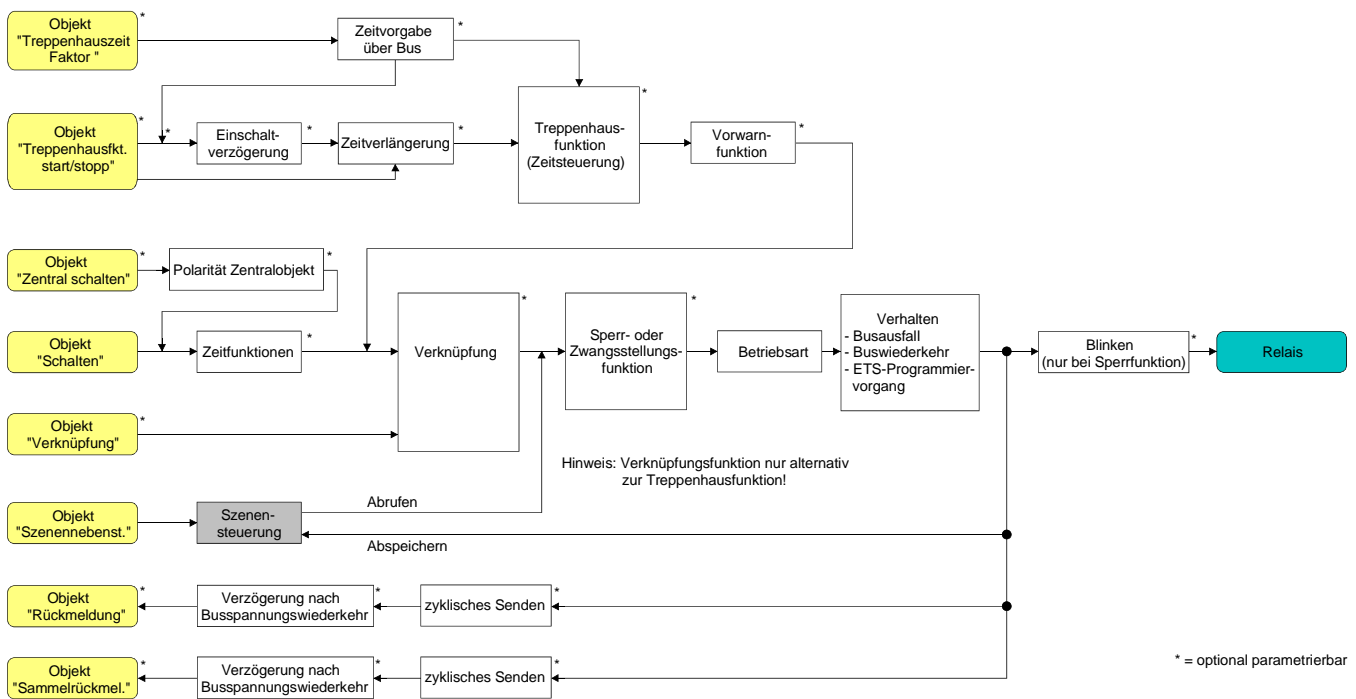
Fig. 15: Funktionsschaltbild der Szenenfunktion
