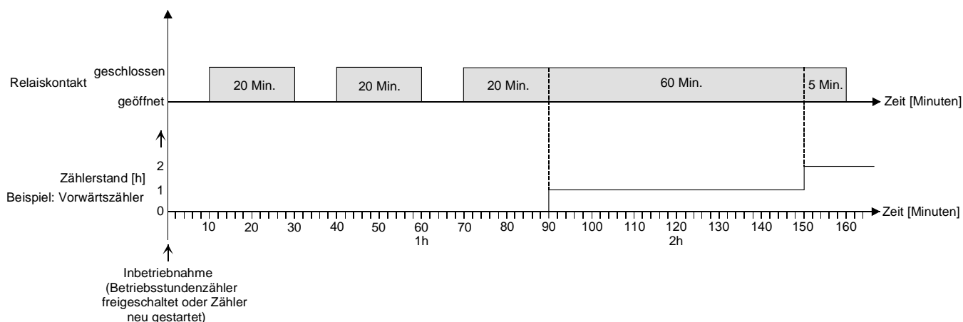
Fig. 16: Funktionsweise des Betriebsstundenzählers
