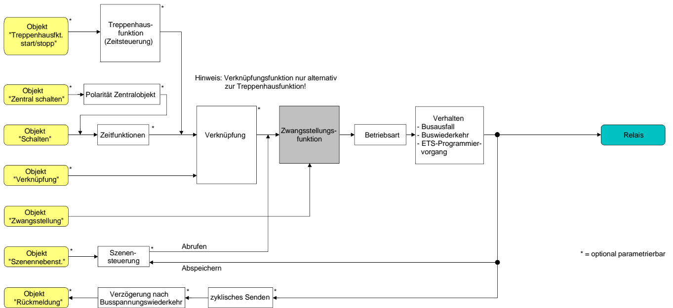
Fig. 18: Funktionsschaltbild der Zwangsstellungsfunktion
