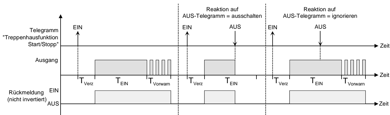
Fig. 12: Ausschaltverhalten der Treppenhausfunktion
