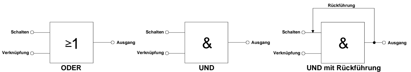
Fig. 20: Verknüpfungsarten der Verknüpfungsfunktion
