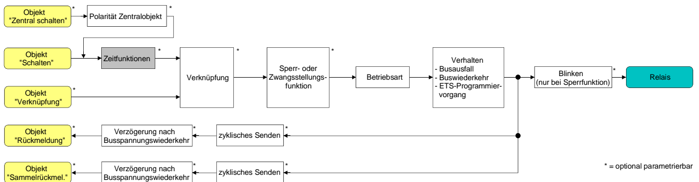
Fig. 9: Funktionsschaltbild der Zeitverzögerungen
