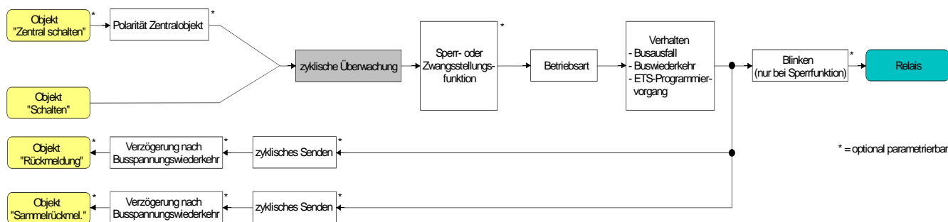
Fig. 8: Funktionsschaltbild der zyklischen Überwachung
