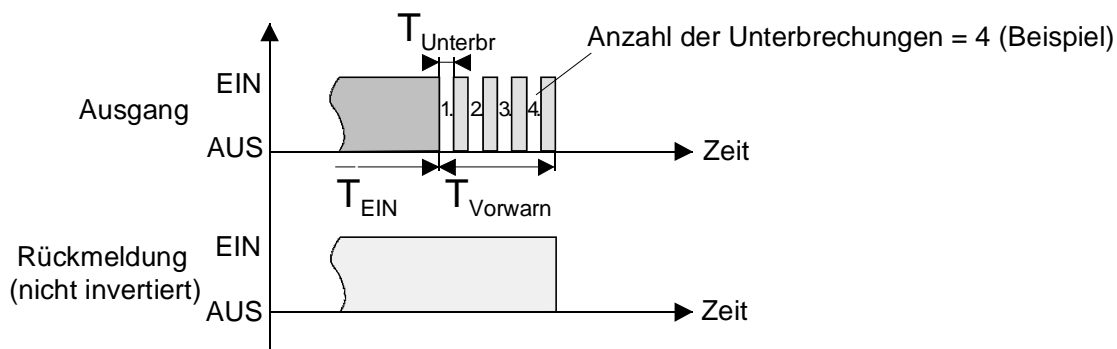
Fig. 13: Die Vorwarnfunktion der Treppenhausfunktion
