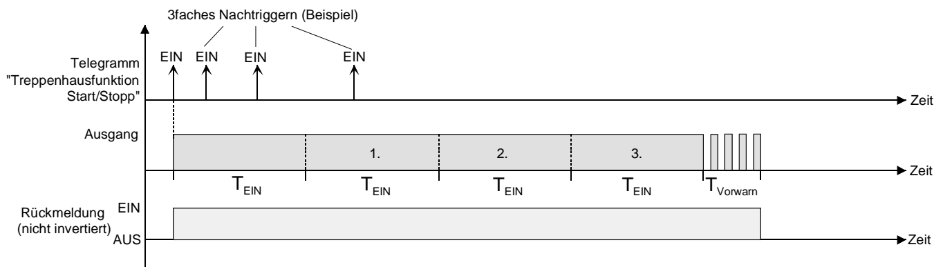
Fig. 14: Zeitverlängerung der Treppenhausfunktion
