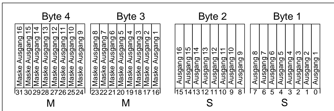
Fig. 5: Struktur des Objektes der Sammelrückmeldung"
