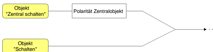
Fig. 4: Funktionsschaltbild "Zentral Schalten"
