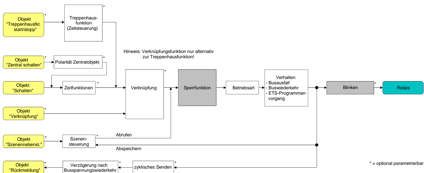
Fig. 17: Funktionsschaltbild der Sperrfunktion
