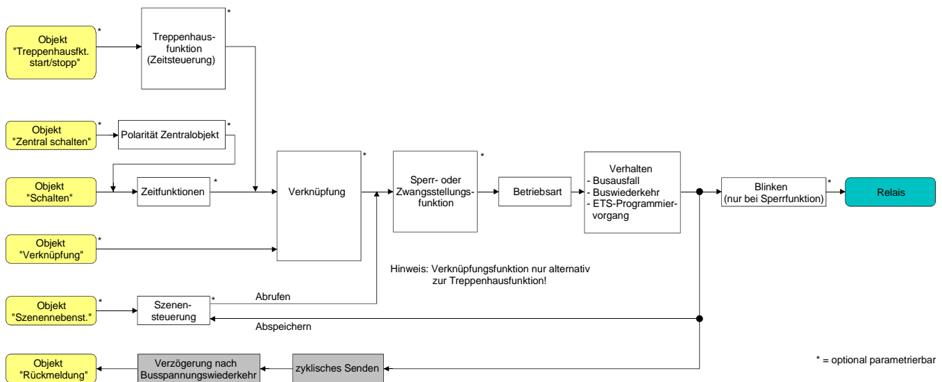
Fig. 7: Funktionsschaltbild der Rückmeldung
