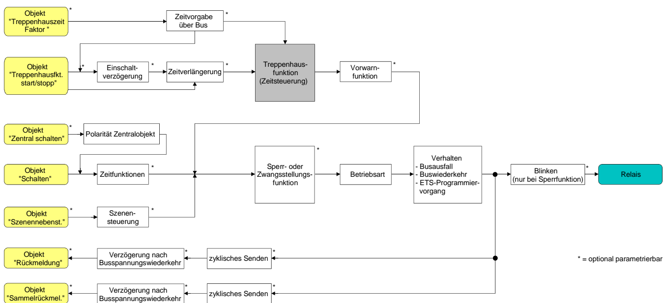
Fig. 10: Funktionsschaltbild der Treppenhausfunktion
