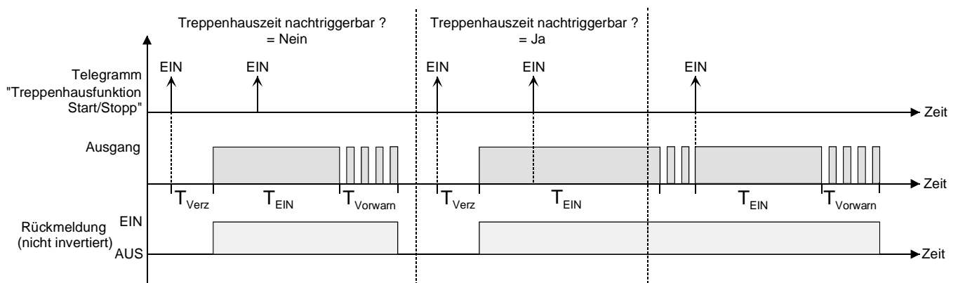
Fig. 11: Einschaltverhalten der Treppenhausfunktion
