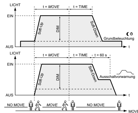
Fig. 2 Grundbeleuchtung / Ausschaltvorwarnung
