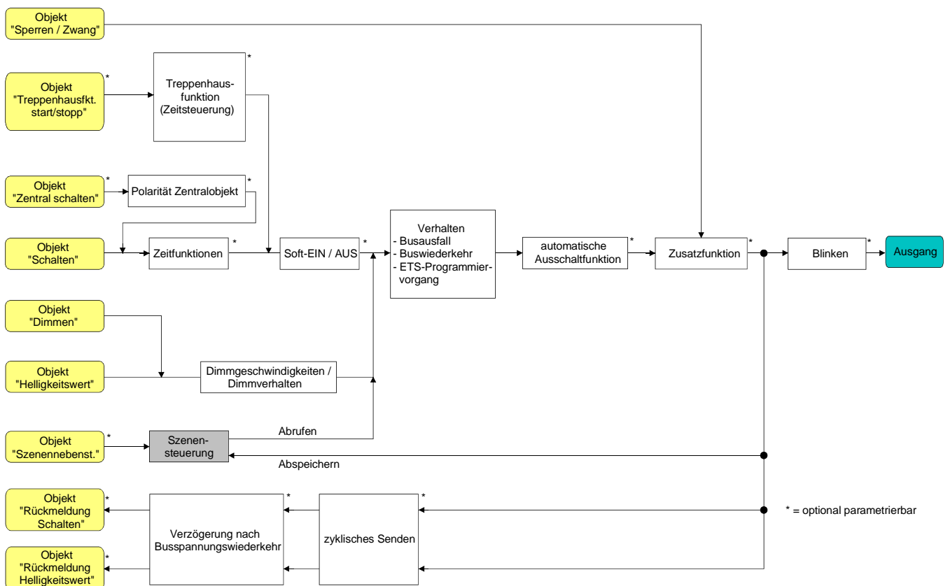
Fig. 20: Funktionsschaltbild der Szenenfunktion
