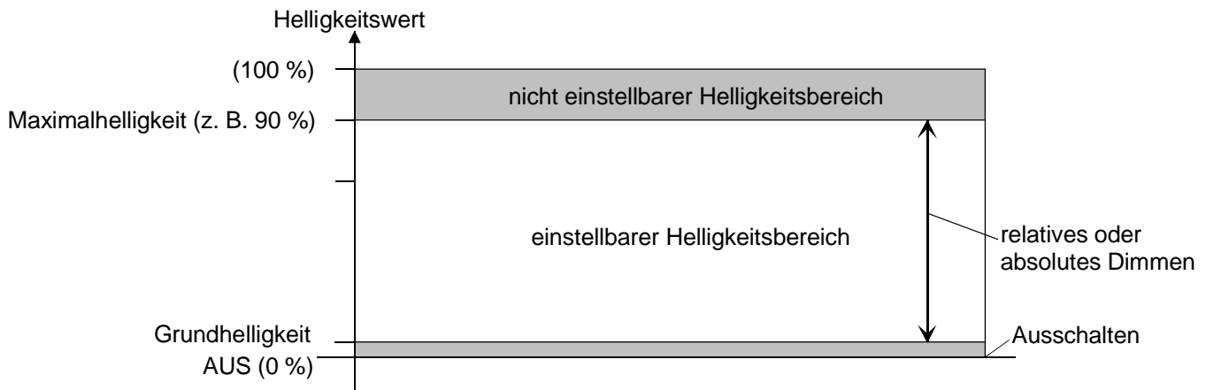
Fig. 24: Einstellbarer Helligkeitsbereich beim Dimmen (Beispiel)
