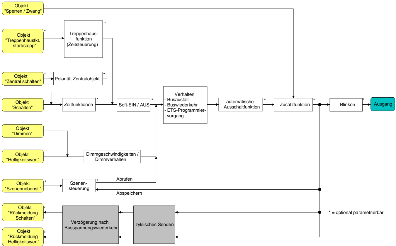
Fig. 6: Funktionsschaltbild der Rückmeldungen
