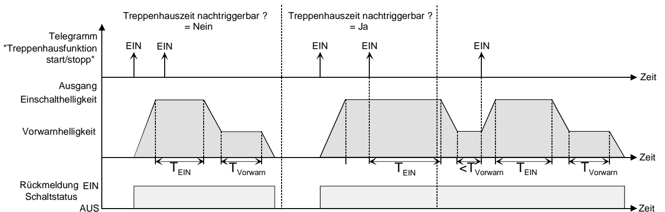
Fig. 14: Einschaltverhalten der Treppenhausfunktion mit Soft-Funktionen (als Beispiel mit Minimalhelligkeit = 0 %)
