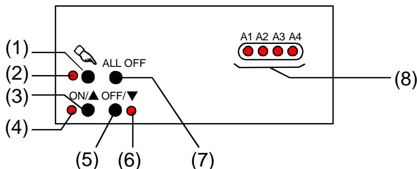
Fig. 3: Bedien- und Anzeigeelemente der Handbedienung
