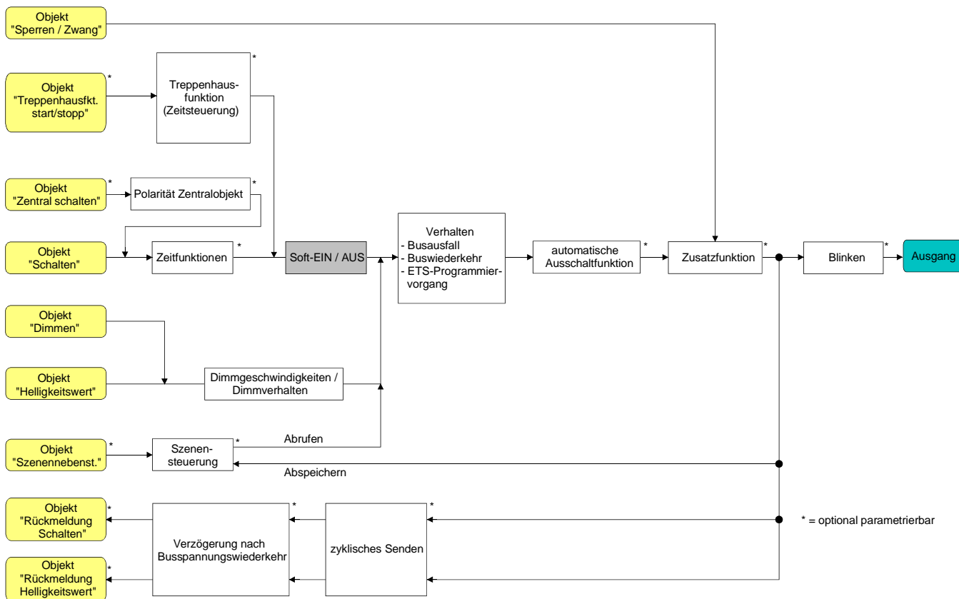
Fig. 9: Funktionsschaltbild der Soft-Funktionen
