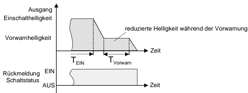
Fig. 18: Die Vorwarnfunktion der Treppenhausfunktion mit Soft-AUS-Funktion (als Beispiel mit Minimalhelligkeit = 0 %)
