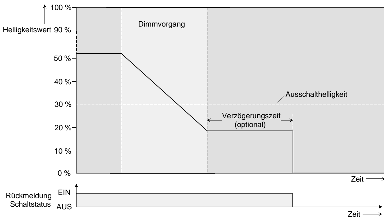
Fig. 10: Dimm- und Schaltverhalten der automatischen Ausschaltfunktion
