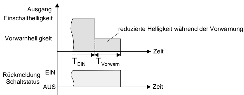
Fig. 17: Die Vorwarnfunktion der Treppenhausfunktion ohne Soft-AUS-Funktion
