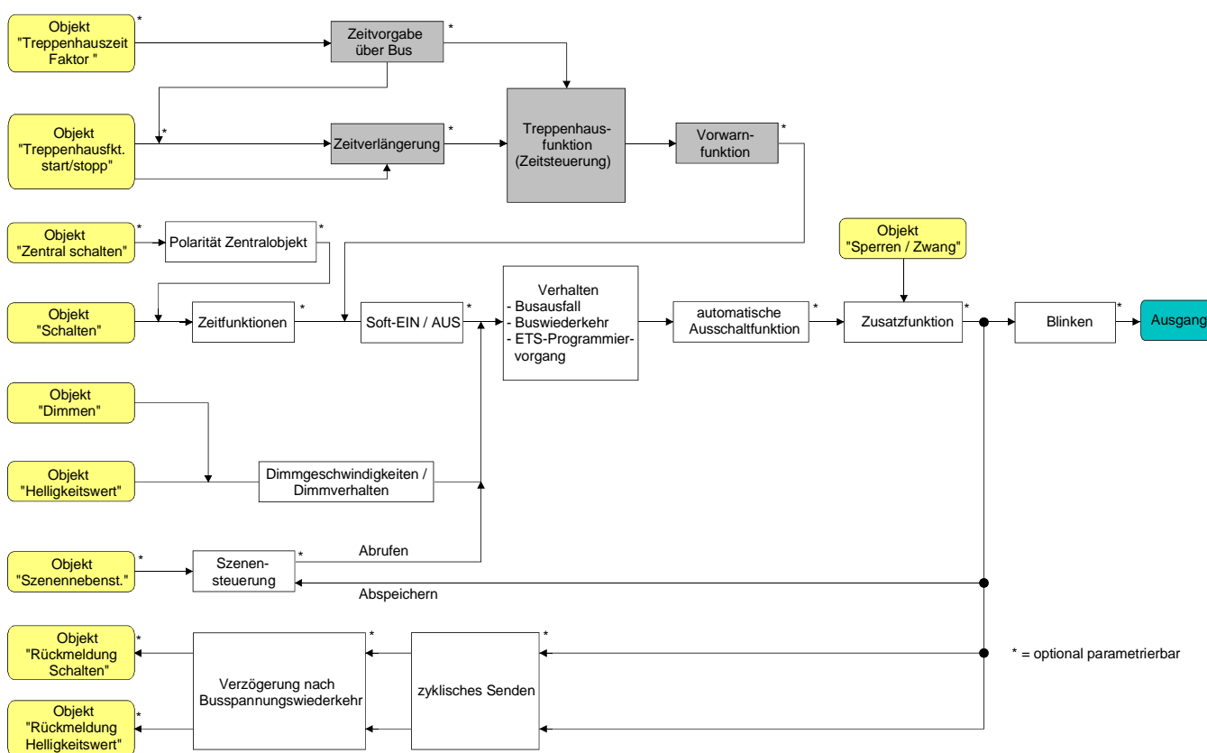
Fig. 12: Funktionsschaltbild der Treppenhausfunktion
