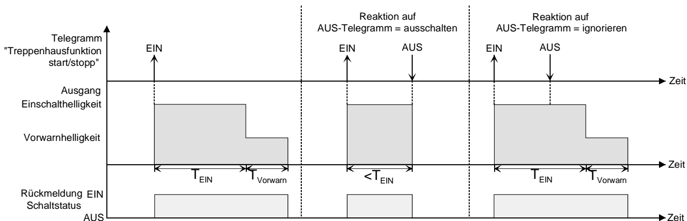
Fig. 15: Ausschaltverhalten der Treppenhausfunktion ohne Soft-Funktionen
