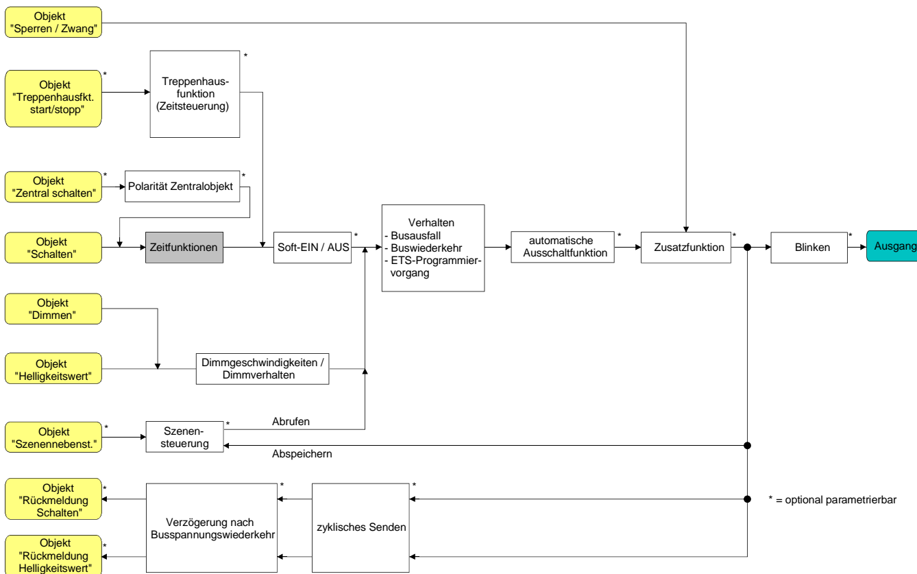
Fig. 7: Funktionsschaltbild der Zeitverzögerungen
