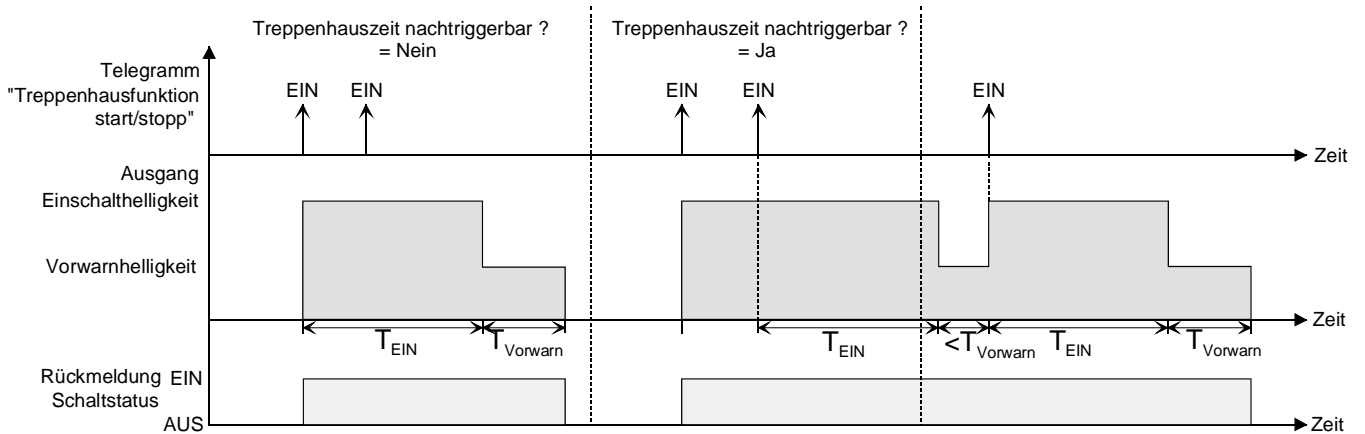
Fig. 13: Einschaltverhalten der Treppenhausfunktion ohne Soft-Funktionen
