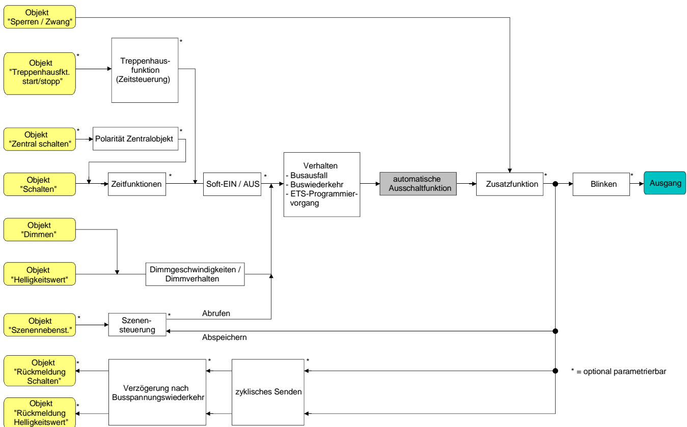
Fig. 11: Funktionsschaltbild der automatischen Ausschaltfunktion
