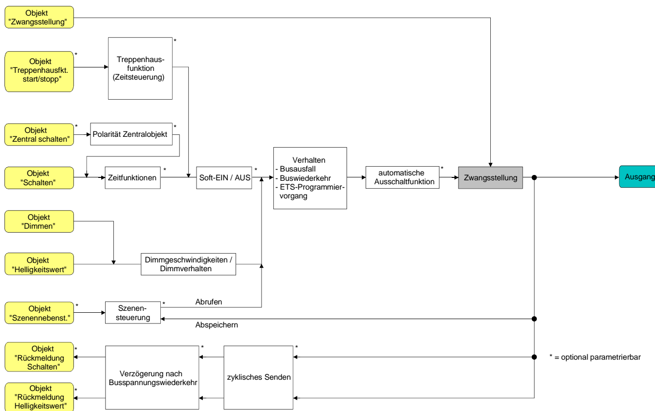
Fig. 23: Funktionsschaltbild der Zwangsstellungsfunktion
