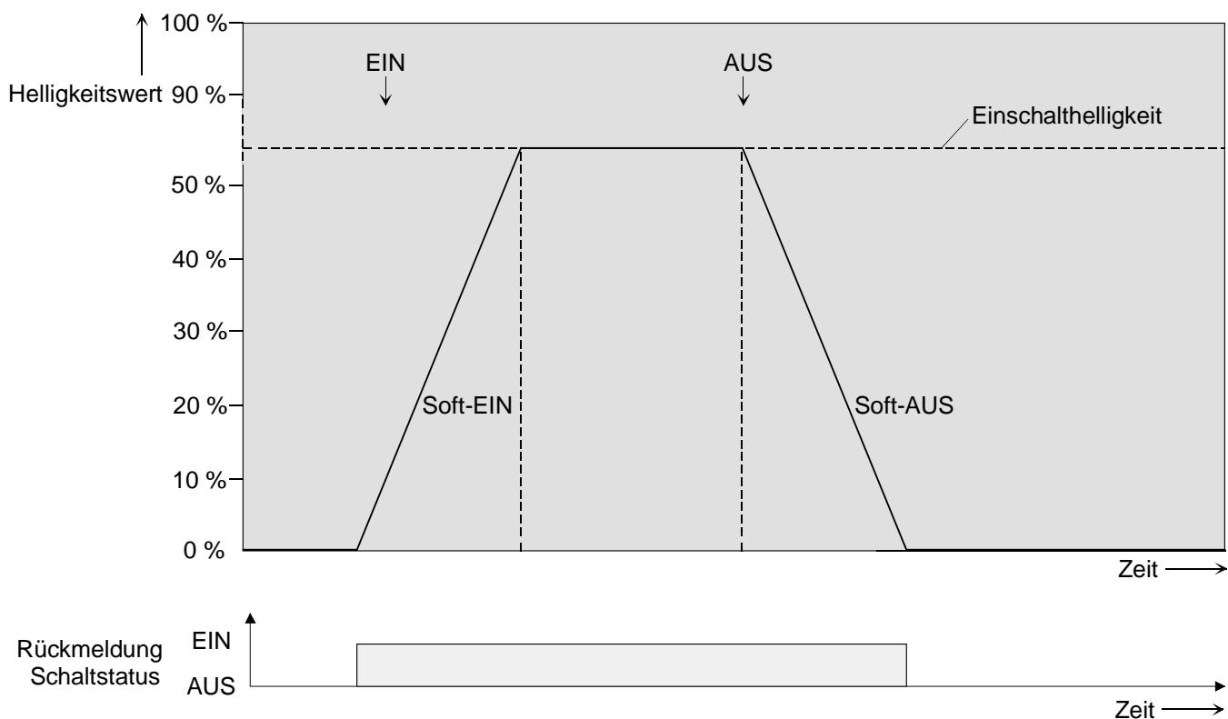
Fig. 8: Dimmverhalten der Soft-EIN/AUS-Funktionen (als Beispiel)
