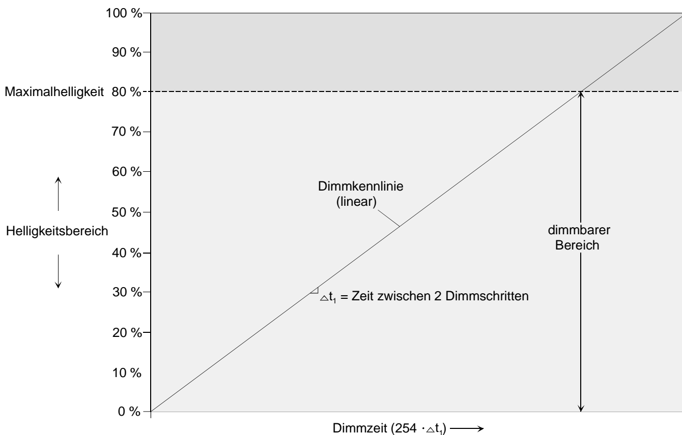
Fig. 25: Lineare Dimmkennlinie als Beispiel mit Maximalhelligkeit < 100 %
