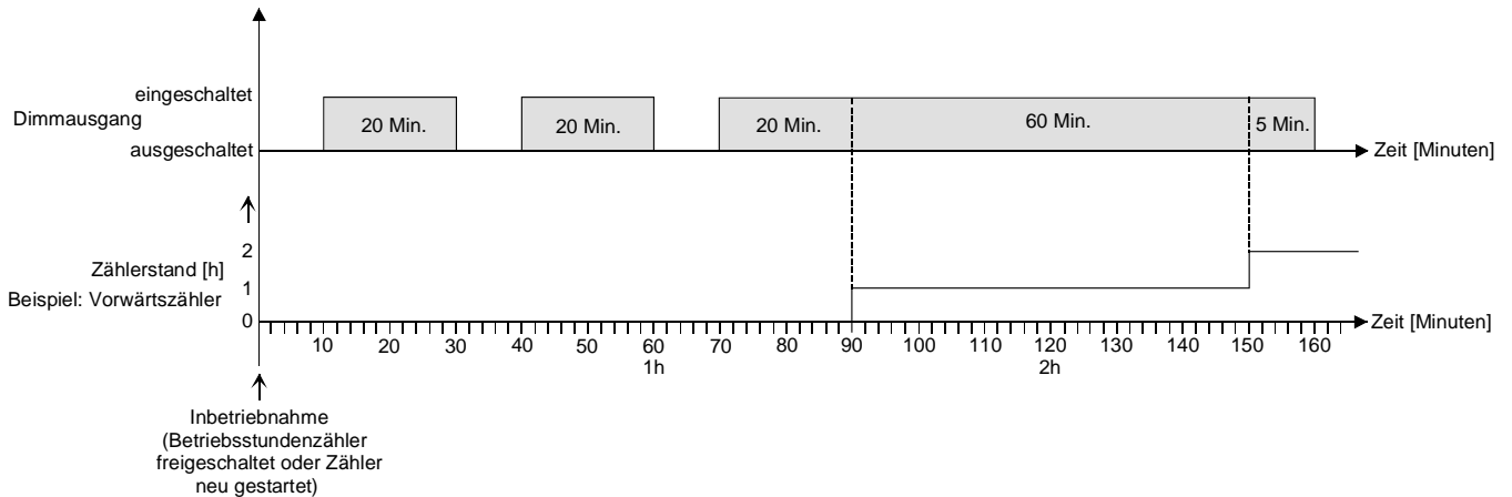
Fig. 21: Funktionsweise des Betriebsstundenzählers
