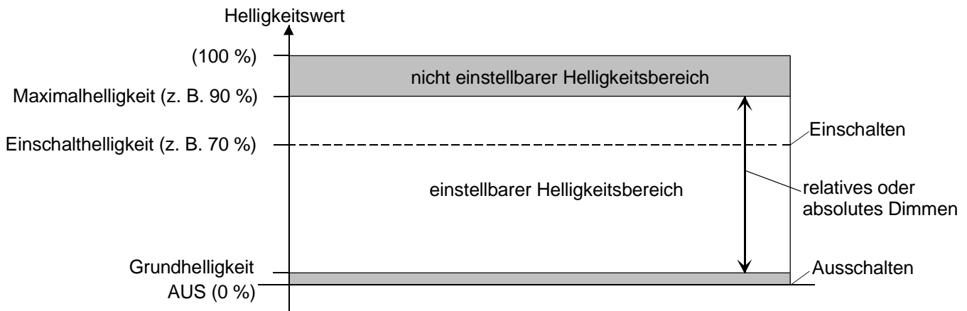
Fig. 5: Beispiel eines Helligkeitsbereiches mit Einschalthelligkeit eines Dimmausgangs
