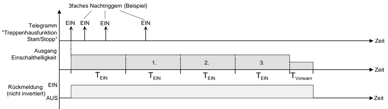
Fig. 19: Zeitverlängerung der Treppenhausfunktion
