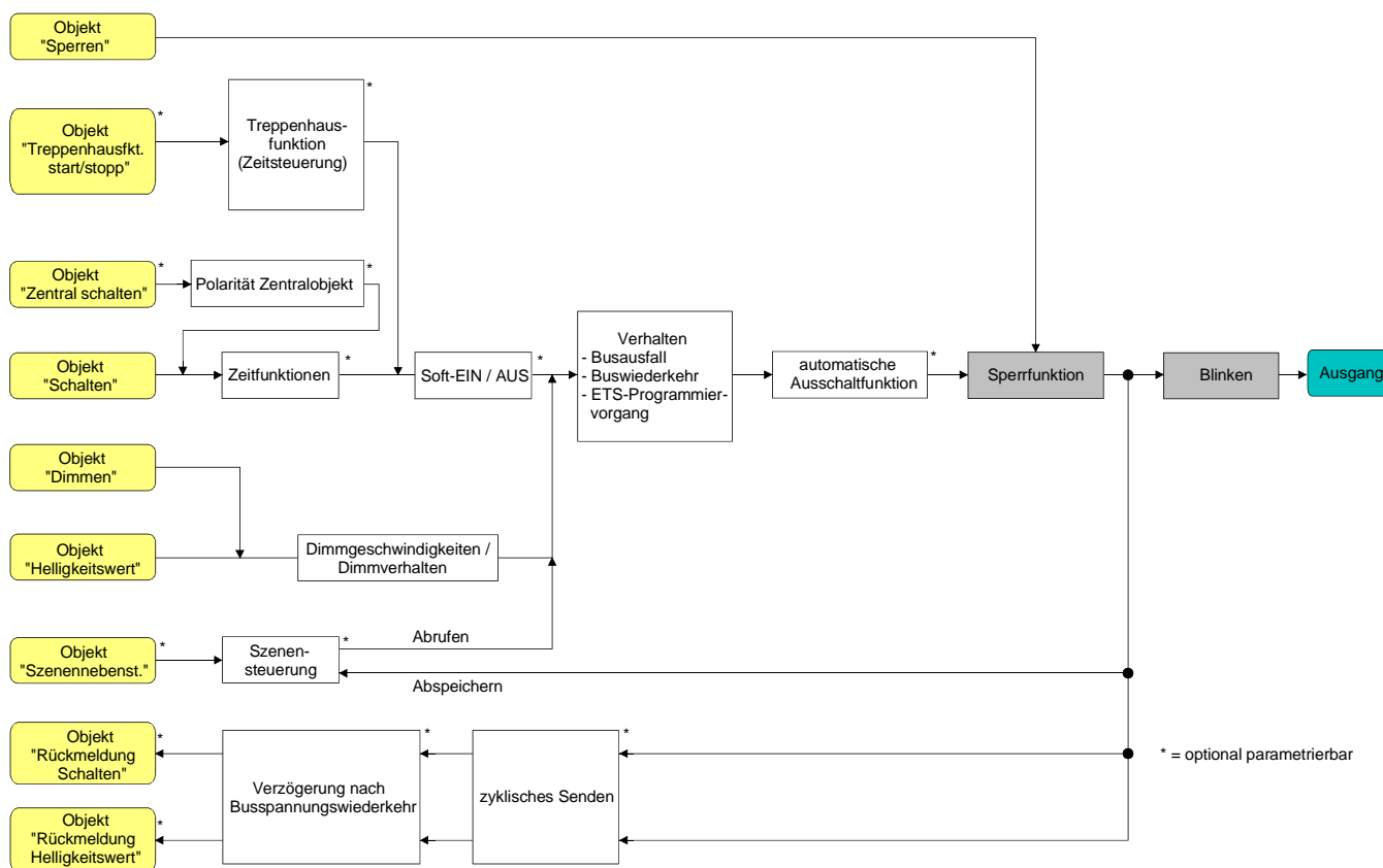
Fig. 22: Funktionsschaltbild der Sperrfunktion
