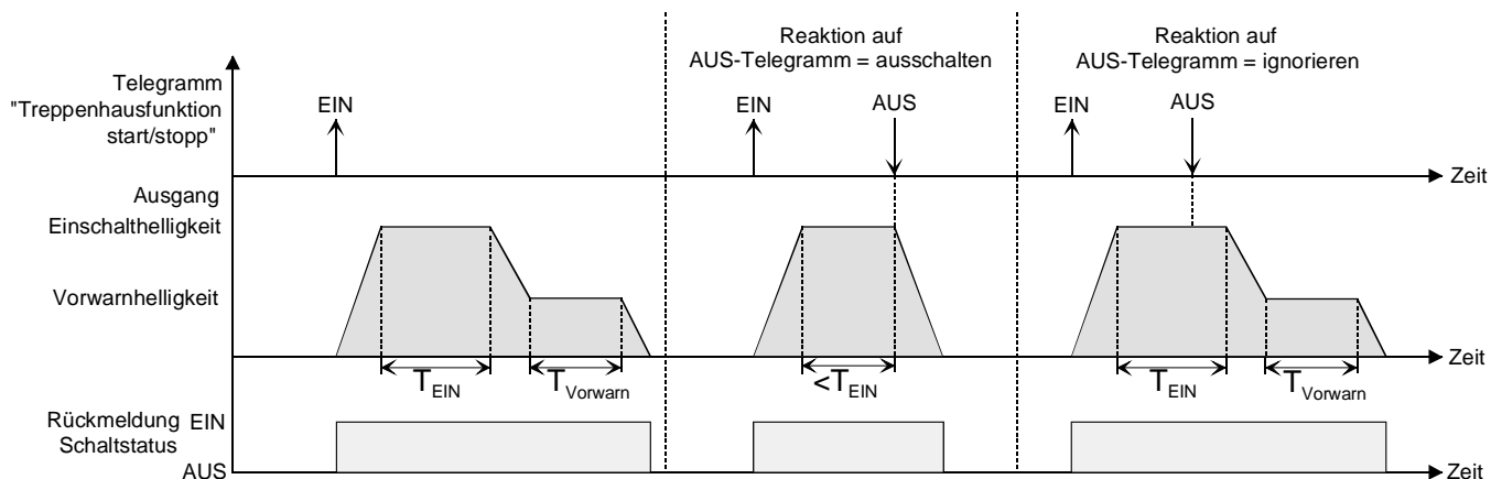
Fig. 16: Ausschaltverhalten der Treppenhausfunktion mit Soft-Funktionen (als Beispiel mit Minimalhelligkeit = 0 %)
