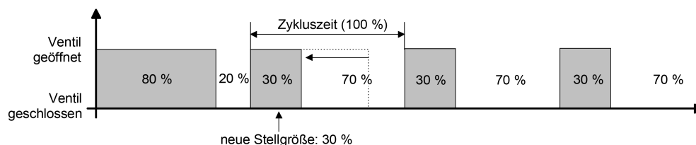
Bild 7: Beispiel einer Stellgrößenänderung 80 % -> 30 % während Öffnungsphase des Ventils
