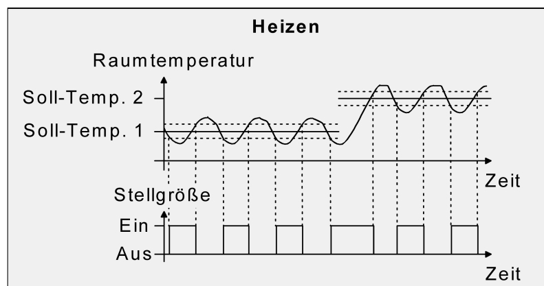
Bild 28: 2-Punkt-Regelung für Einzelbetriebsart "Heizen"
