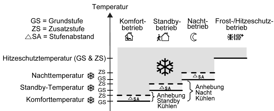
Bild 38: Solltemperaturen in der Betriebsart "Grund- und Zusatzkühlen"
