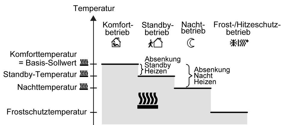
Bild 35: Solltemperaturen in der Betriebsart "Heizen"
