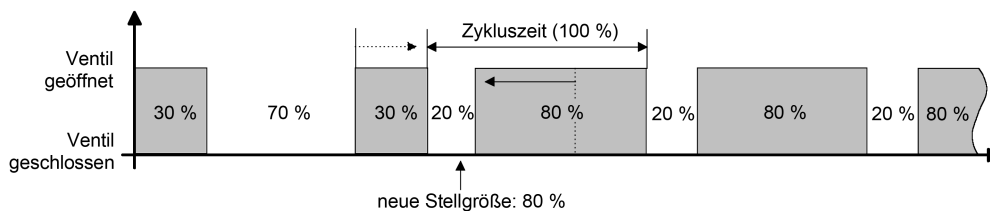
Bild 11: Beispiel einer Stellgrößenänderung 30 % -> 80 % während Schließphase des Ventils
