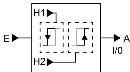
Bild 47: Grenzwertschalter
