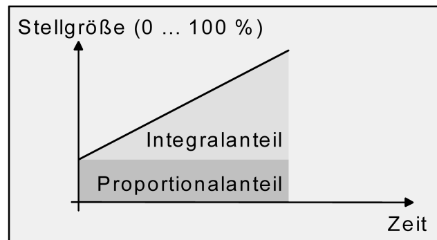
Bild 26: Stetige PI-Regelung
