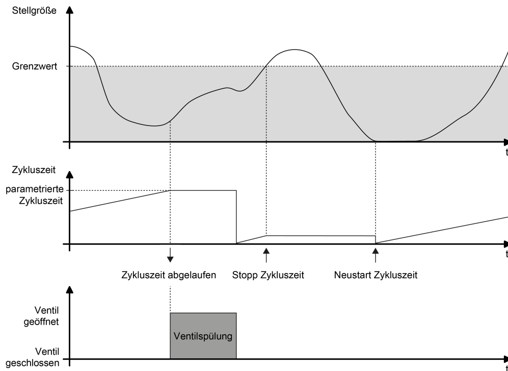
Bild 23: Beispiel eines minimalen Stellgrößen-Grenzwerts für die intelligente Ventilspülung
