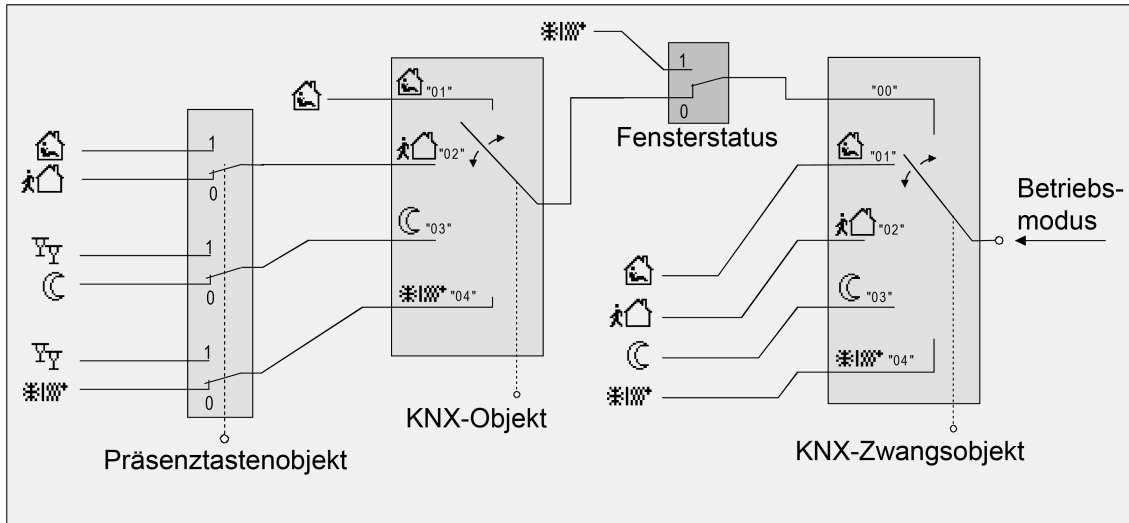
Bild 33: Betriebsmodusumschaltung durch KNX Objekt mit Präsenztaste
