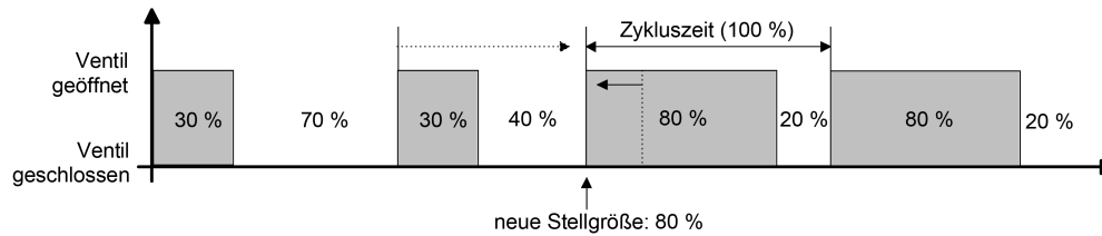
Bild 12: Beispiel einer Stellgrößenänderung 30 % -> 80 % während Öffnungsphase des Ventils (Öffnungsphase zu lang)
