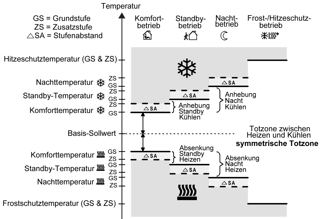
Bild 41: Solltemperaturen in der Betriebsart "Grund- und Zusatzheizen und -kühlen" mit symmetrischer Totzone
