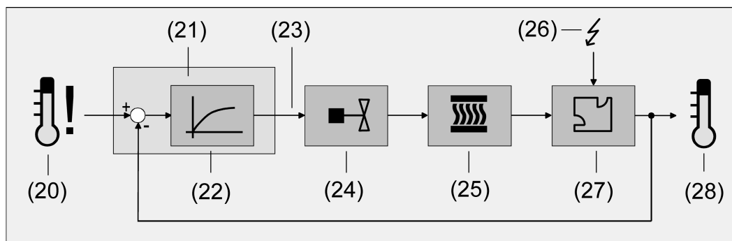
Bild 25: Regelstrecke einer Einzelraum-Temperaturregelung
