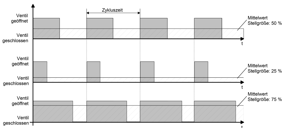
Bild 6: Resultierender Mittelwert durch variables Tastverhältnis bei einer Pulsweitenmodulation
