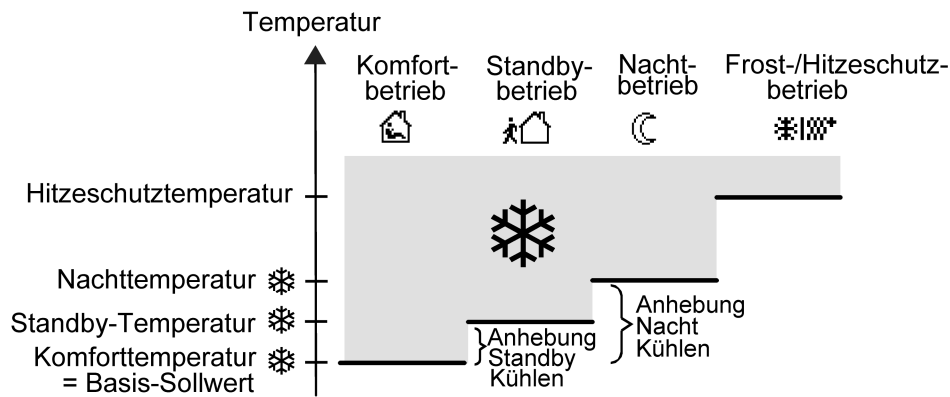
Bild 37: Solltemperaturen in der Betriebsart "Kühlen"
