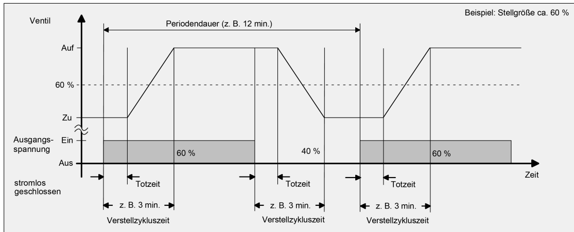
Bild 14: Idealisierter Verlauf des Ventilhubes exemplarisch dargestellt für eine Zykluszeit > 2 \times Verstellzykluszeit
