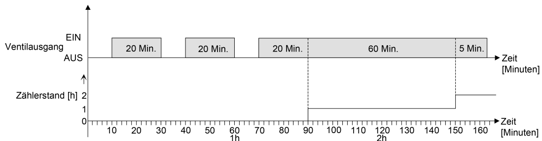
Bild 24: Funktionsweise des Betriebsstundenzählers (am Beispiel eines Vorwärtszählers)
