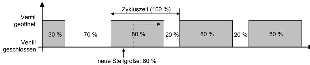
Bild 10: Beispiel einer Stellgrößenänderung 30 % -> 80 % während Öffnungsphase des Ventils
