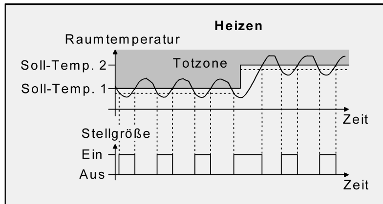
Bild 30: 2-Punkt-Regelung für Mischbetriebsart "Heizen und Kühlen" bei aktivem Heizbetrieb
