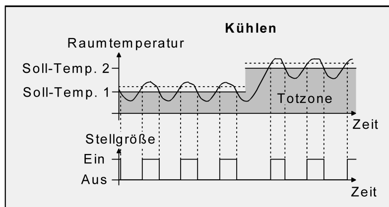
Bild 31: 2-Punkt-Regelung für Mischbetriebsart "Heizen und Kühlen" bei aktivem Kühlbetrieb
