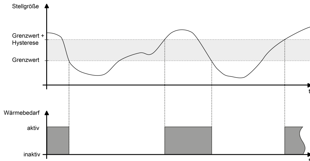
Bild 4: Wärmebedarfsinformation mit beispielhaftem Stellgrößenverlauf
