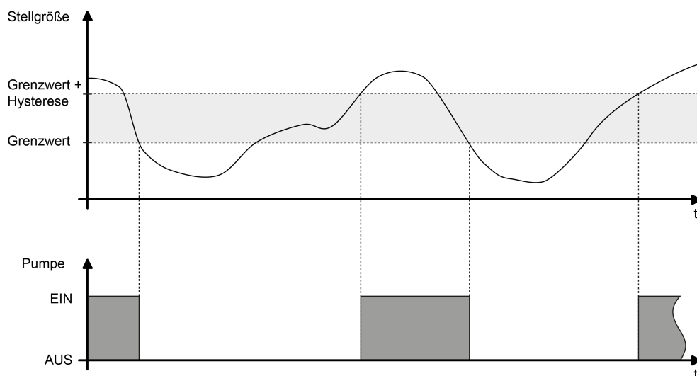
Bild 5: Pumpensteuerung mit beispielhaftem Stellgrößenverlauf
