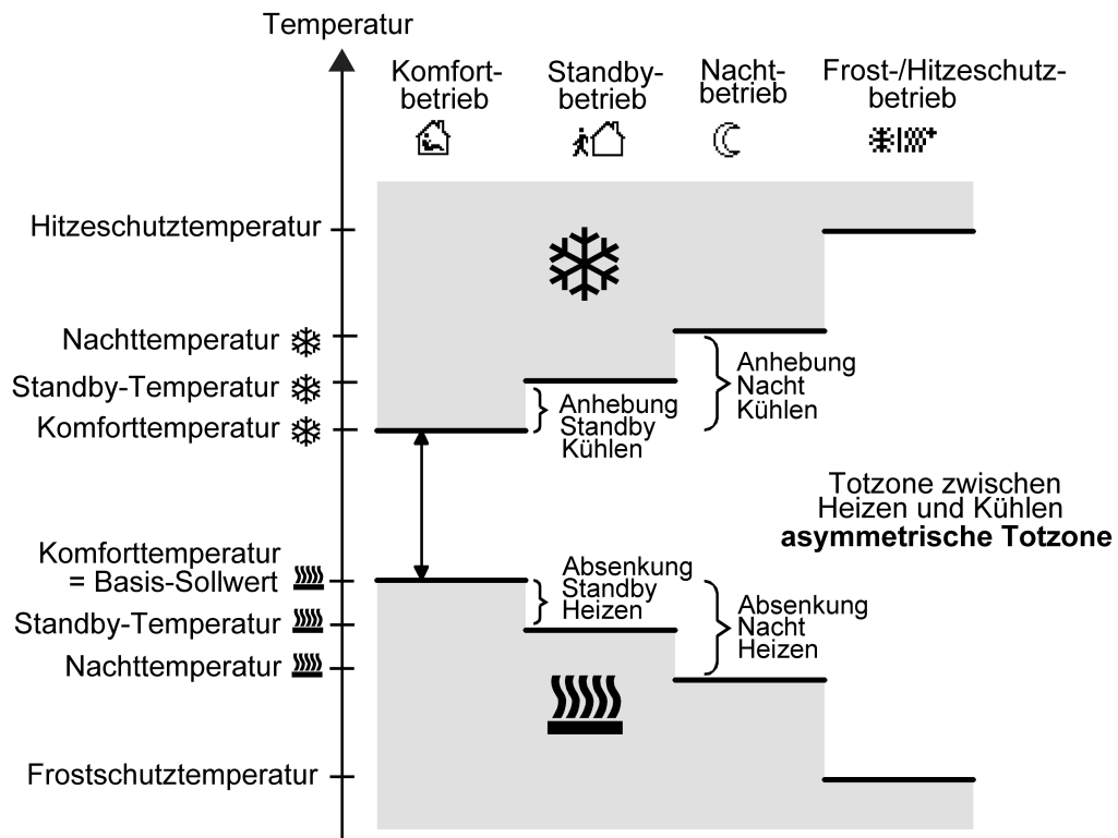
Bild 40: Solltemperaturen in der Betriebsart "Heizen und Kühlen" mit asymmetrischer Totzone
