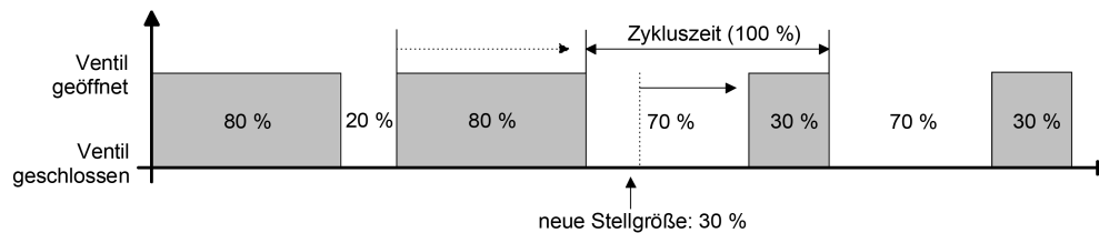
Bild 8: Beispiel einer Stellgrößenänderung 80 % -> 30 % während Schließphase des Ventils
