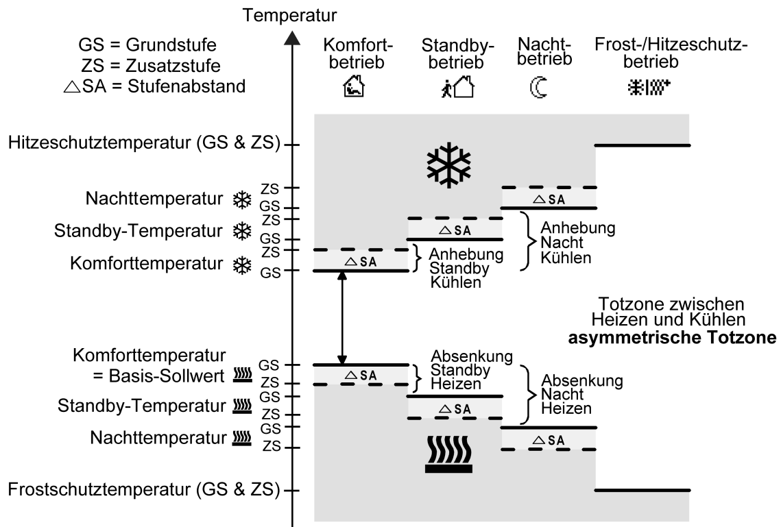
Bild 42: Solltemperaturen in der Betriebsart "Grund- und Zusatzheizen und -kühlen" mit asymmetrischer Totzone
