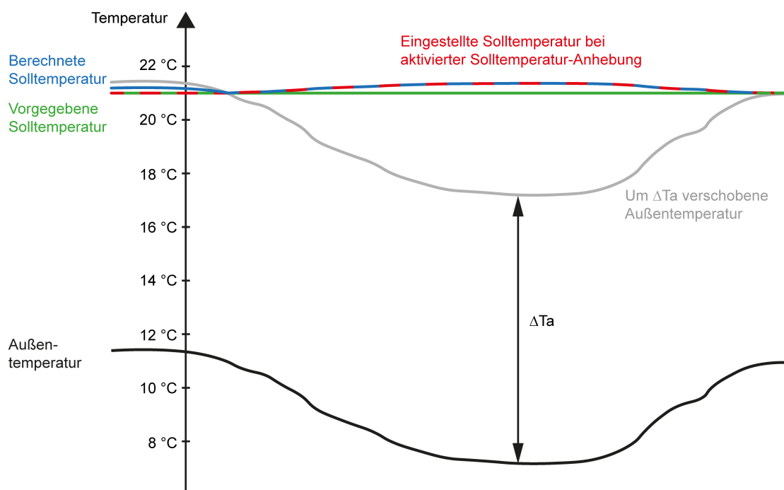
Bild 43: Beispiel zur Winterkompensation
