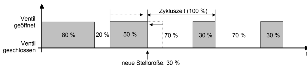
Bild 9: Beispiel einer Stellgrößenänderung 80 % -> 30 % während Öffnungsphase des Ventils (Öffnungsphase zu lang)
