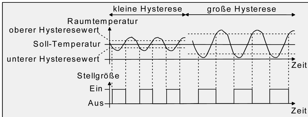
Bild 32: Auswirkungen der Hysterese auf das Schaltverhalten der Stellgröße einer 2-Punkt-Regelung
