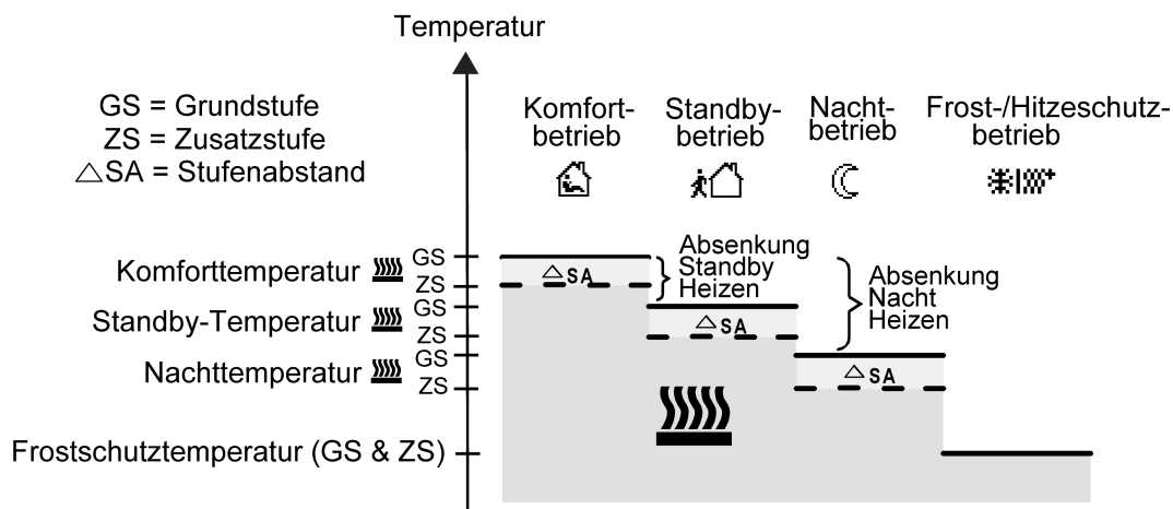
Bild 36: Solltemperaturen in der Betriebsart "Grund- und Zusatzheizen"
