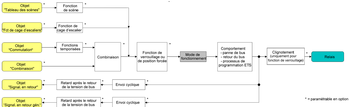
Fig. 6: Schéma de câblage fonctionnel "Mode de fonctionnement"
