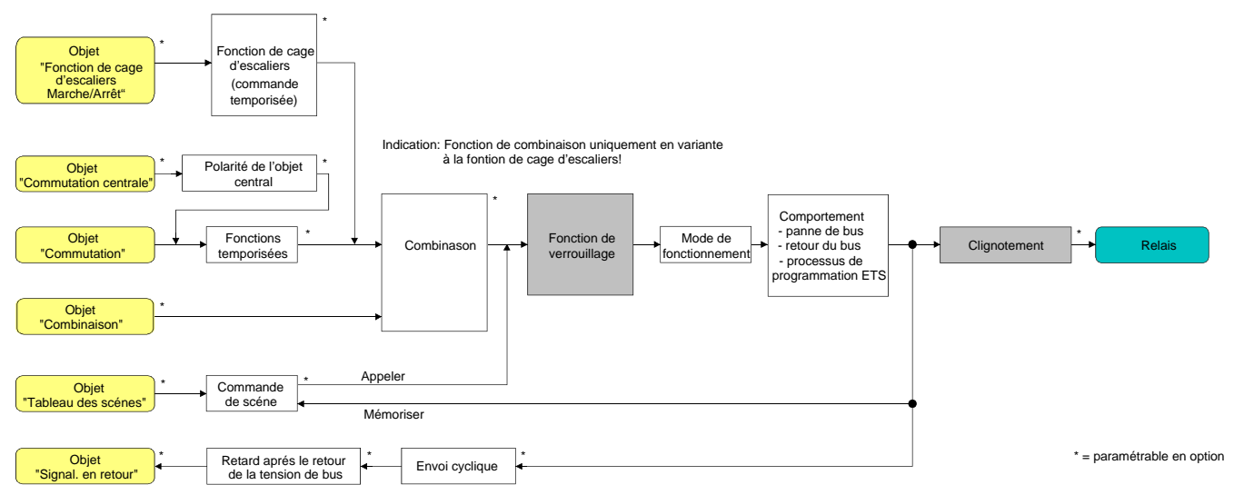
Fig. 17: Schéma de câblage fonctionnel de la fonction de verrouillage
