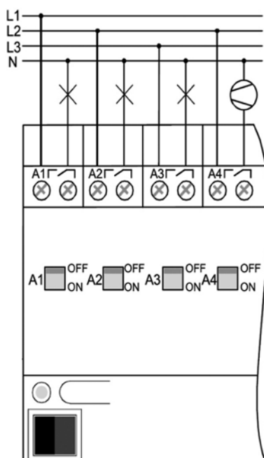
Fig. 1: Raccordement électrique
