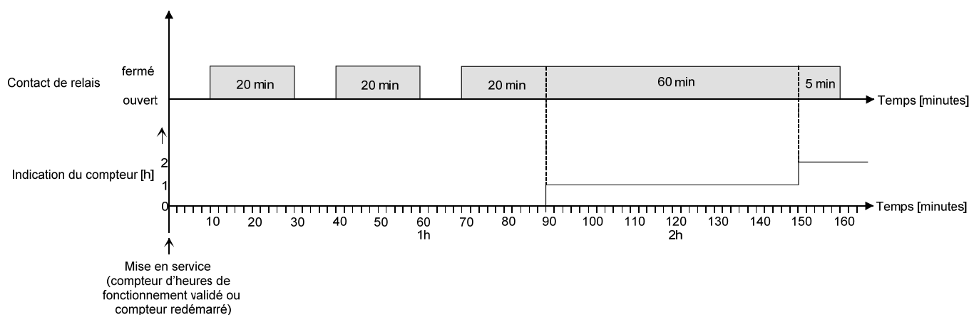
Fig. 16: Mode de fonctionnement du compteur d'heures de fonctionnement
