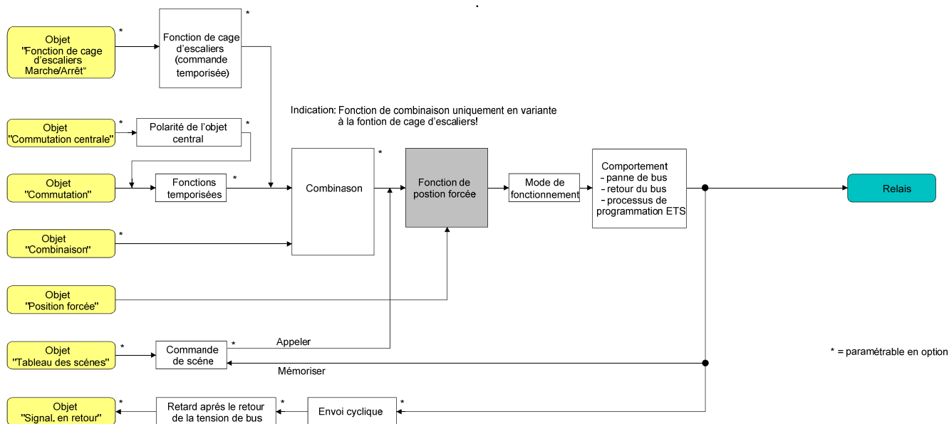
Fig. 18: Schéma de câblage fonctionnel de la fonction de position forcée
