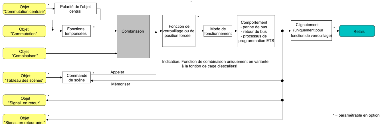
Fig. 19: Schéma de câblage fonctionnel de la fonction de combinaison
