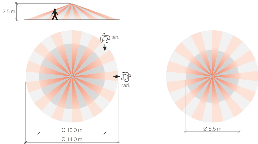
Erfassungsbereich pirios 360 KNX / mit Reduktion
