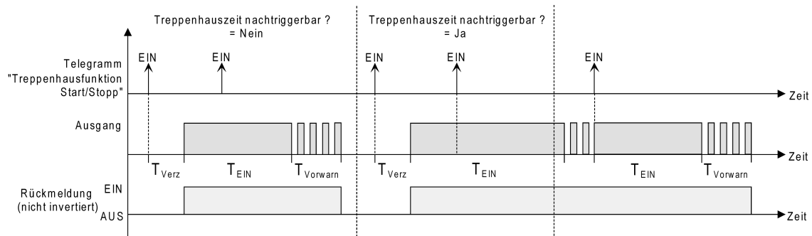
Bild 17: Einschaltverhalten der Treppenhausfunktion
