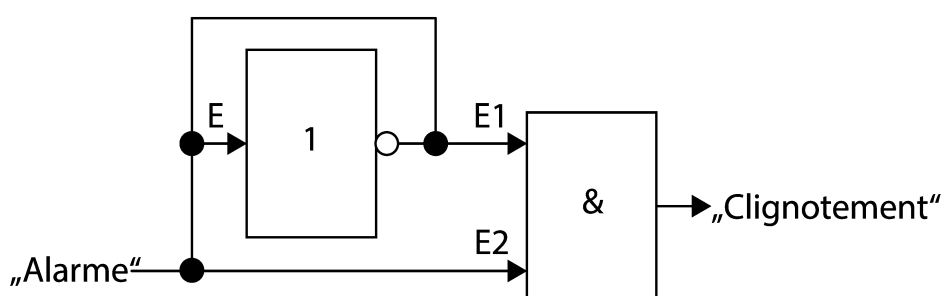
Figure 16: Représentation schématique « clignotement »
