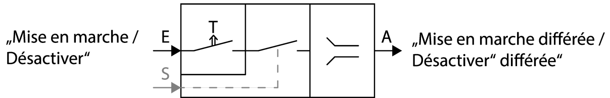
Figure 19: Représentation schématique « Enclenchement et déclenchement temporisés »
