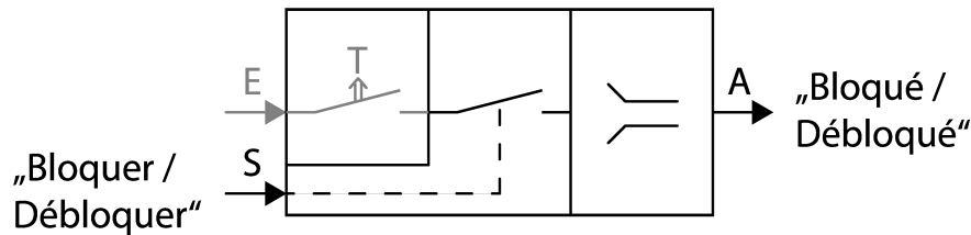
Figure 21: Représentation schématique de la « fonction de blocage »
