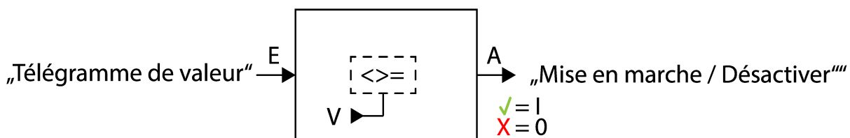
Figure 22: Représentation schématique « Affichage de l'état de la valeur de comparaison »
