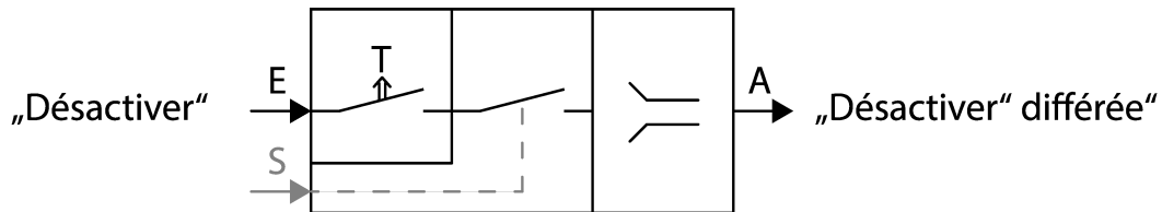
Figure 18: Représentation schématique « Arrêt différé »
