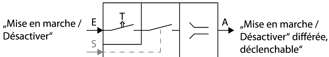
Figure 20: Représentation schématique « fonction cage d'escalier »
