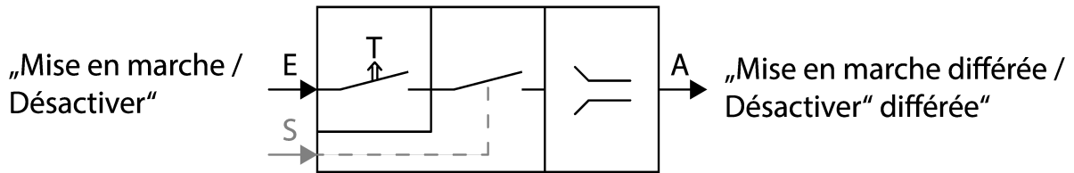
Figure 23: Représentation schématique « Enclenchement et déclenchement temporisés »
