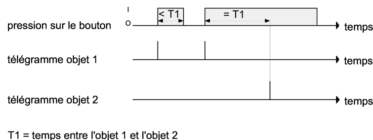
Figure 15: Exemple de concept de commande « Objet 1 et objet 2 »
